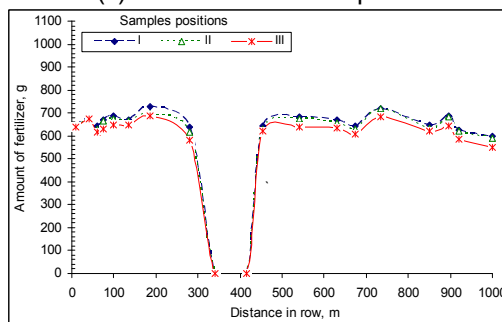
(d) 6.70 km/h forward speed.
